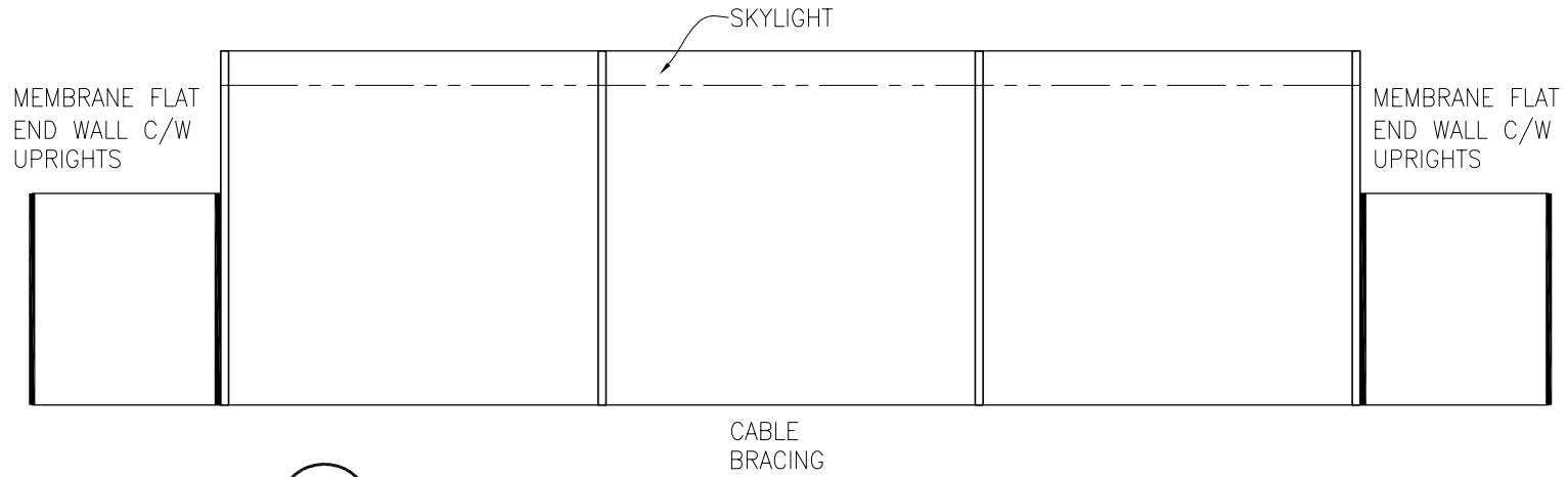
○ ELEVATION 1:125
